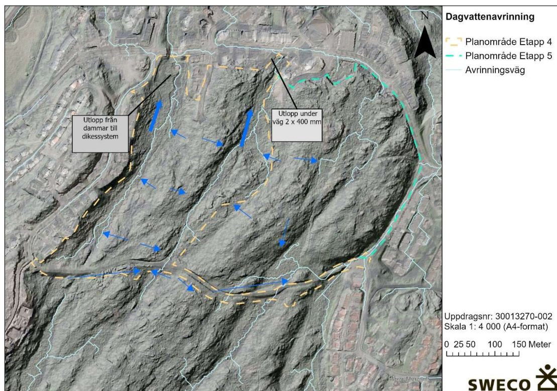
Figur 5. Befintlig dagvattenavrinning innan exploatering (Sweco, 2022).
