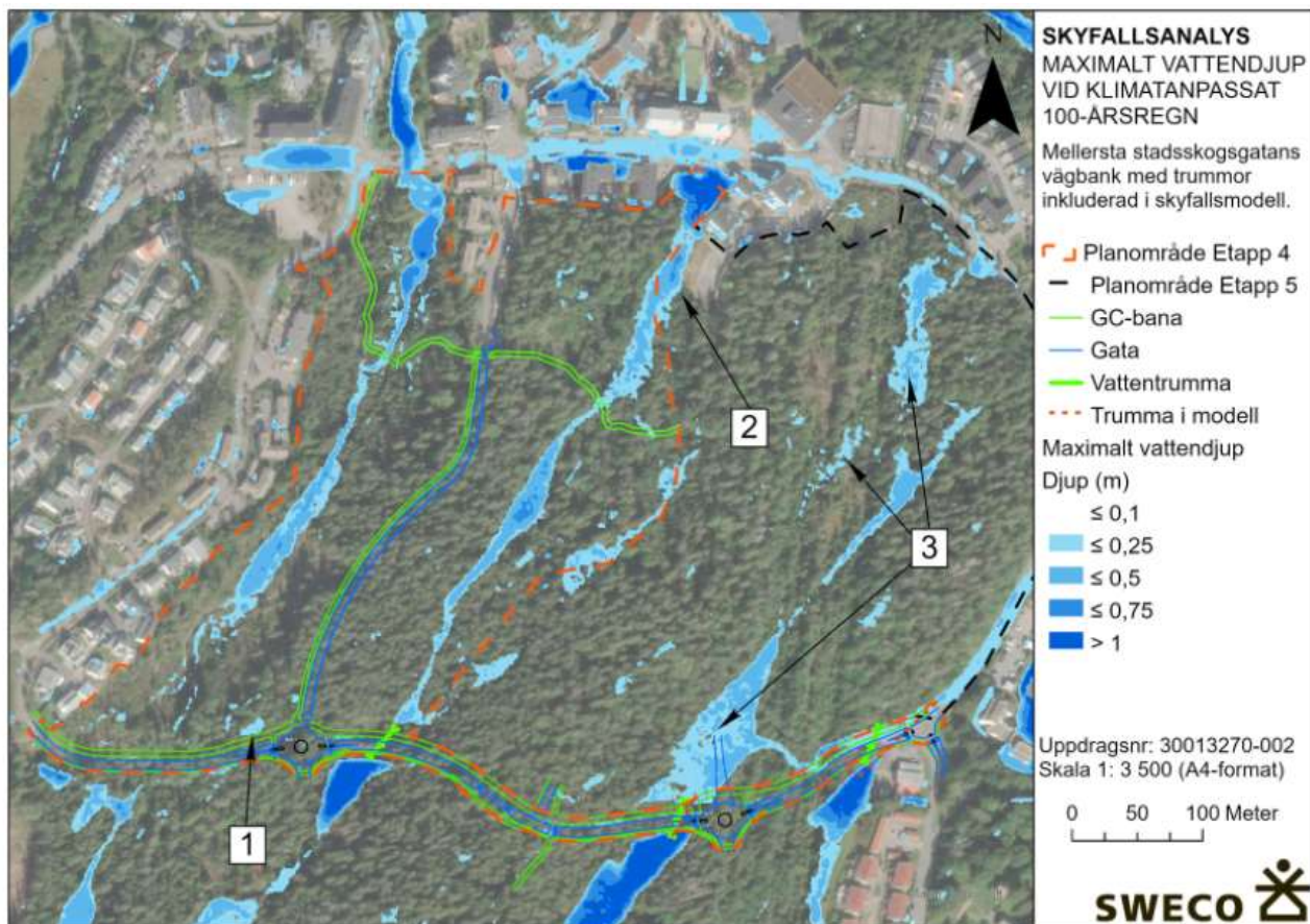
Figur 22. Skyfallsanalys med fokusområden. Blå områden visar på vart vatten vid ett skyfall står samt vid vilket djup (Sweco, 2022).
