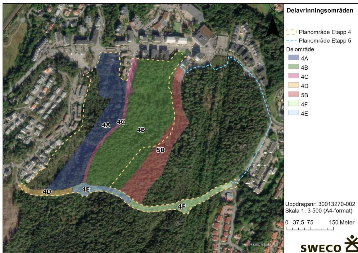
Figur 6 Delområden för avrinning inom planområdet för etapp 4 samt del av etapp 5 (Sweco, 2022).
