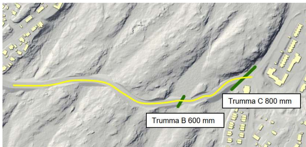
Figur 23. Kulvertar inlagda i skyfallsmodell (Sweco, 2021).
