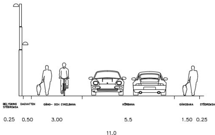
Figur 17. Alternativ utformning Trollskogsgatan (Sweco, 2021-04-13).
