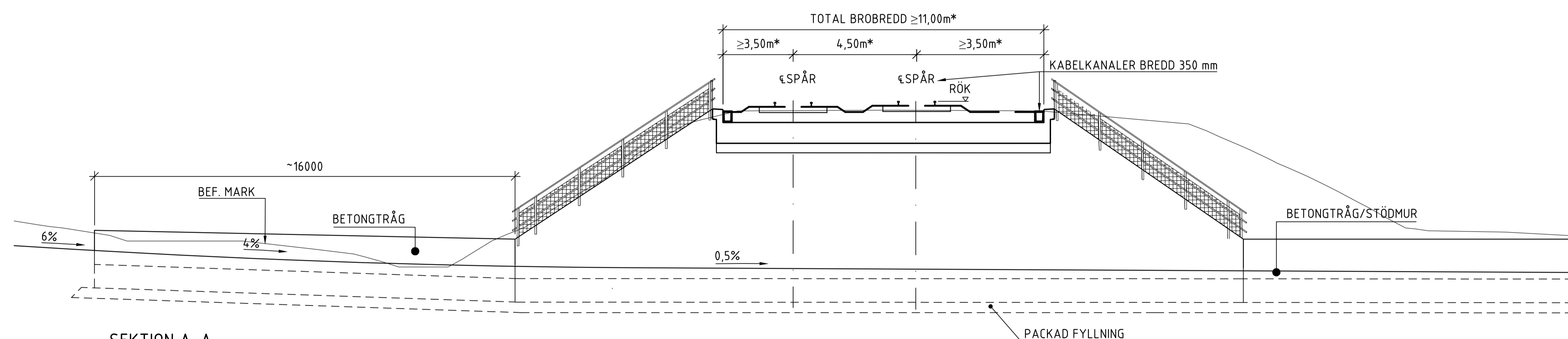
SEKTION A-A 1:100
