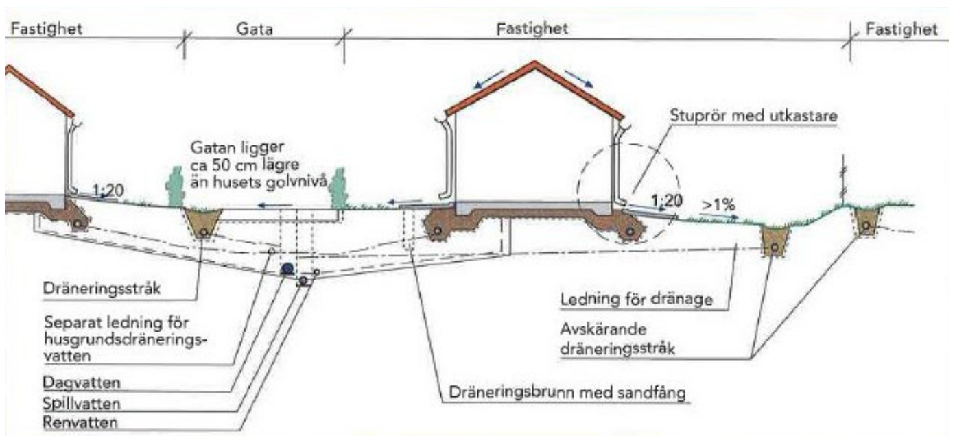
Sektion med föreslagna marklutningar (Cowi, 2021-04-19)
