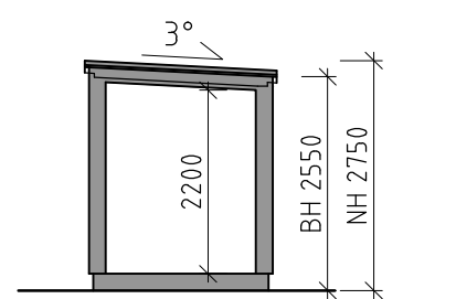
Förråd - Sektion
