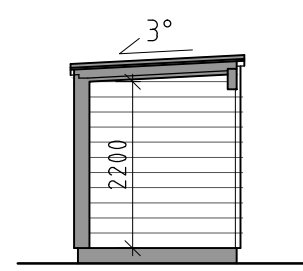
Förråd - Fasad mot nordväst Uteplats - Sektion
