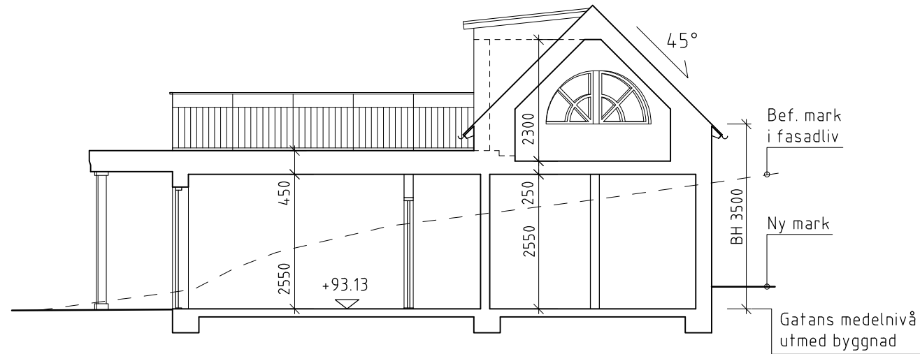
Sektion C-C
