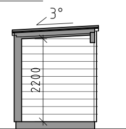
Förråd - Fasad mot norr Uteplats - Sektion
