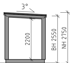
Förråd - Sektion
